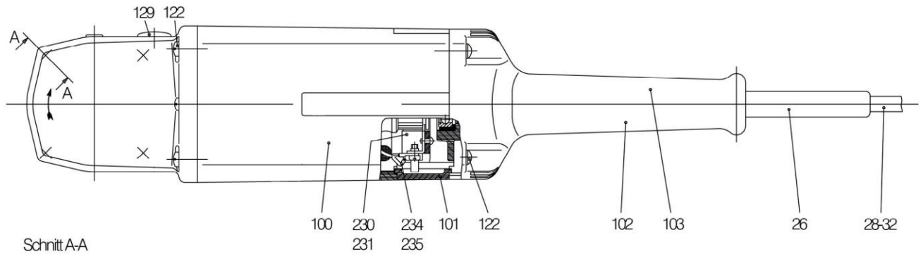
Schnitt A-A
